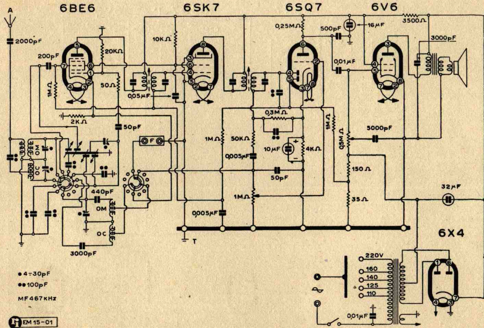
Lo schema elettrico del Mod. PD 14
